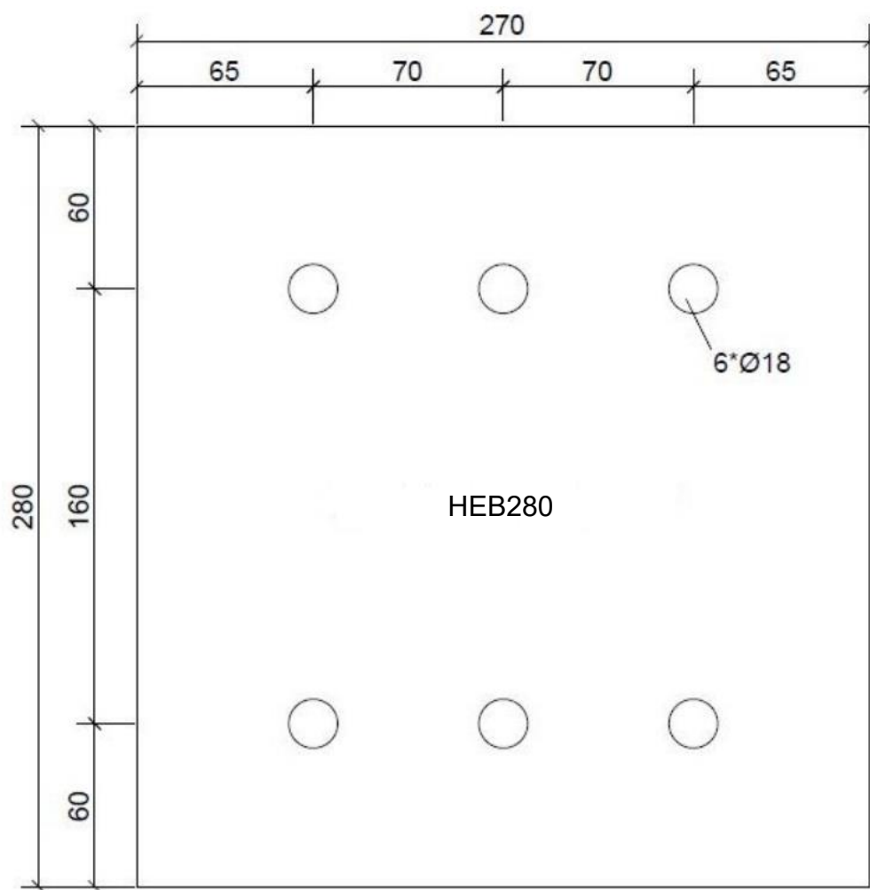
Kopplaat HEB280
