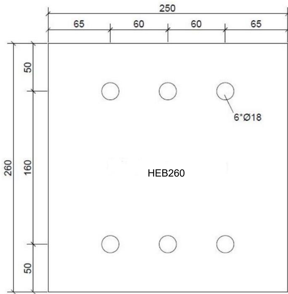
Kopplaat HEB260
